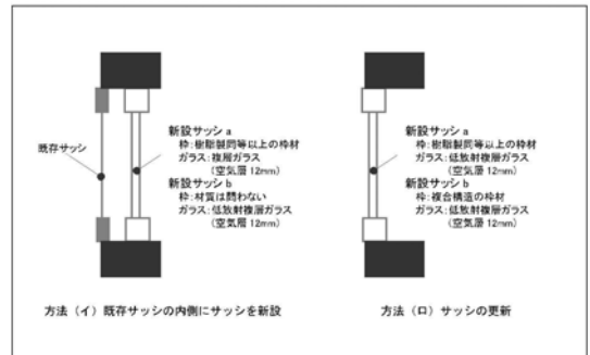
図 3-1-3 熱貫流率U=2.33 [W/(m 2 ·K)]以下の仕様
